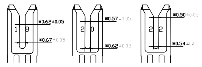
<A型>18#线端子 <B型>20#线端子 <C型>22#线端子
